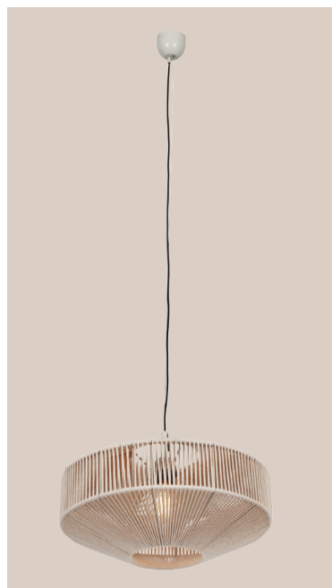
ITEMNO• EQ260004-40 MATERIAL• METAL+ROPE LAMP HOLDER• E27*1 COLOR• BK SIZE• D400*H1200MM
